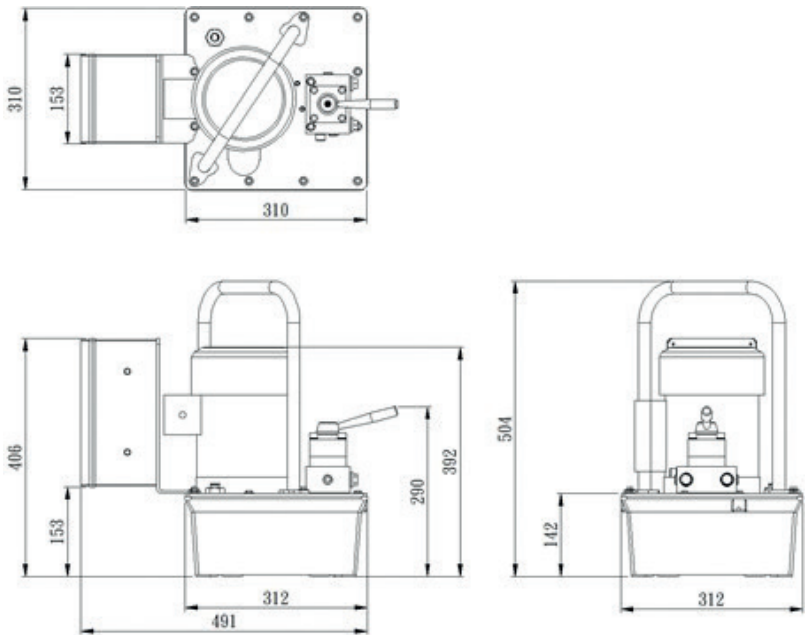
Maßzeichnung EP211
