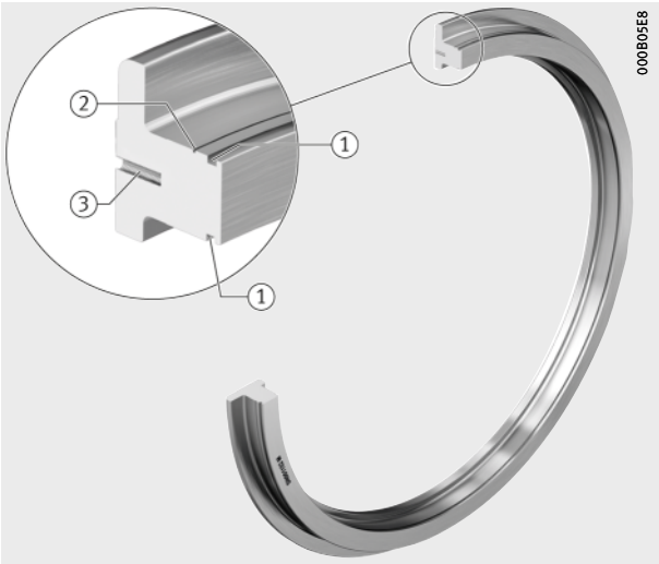
Figura 4 Cilindro anular
