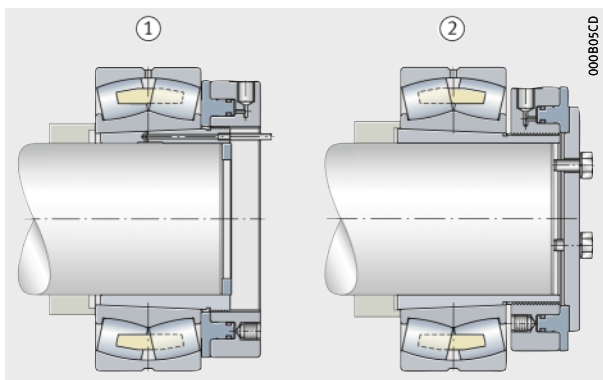
Figura 8 Procedimiento de desmontaje
