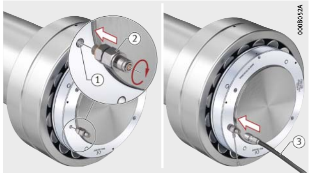
Figura 27 Conexión
