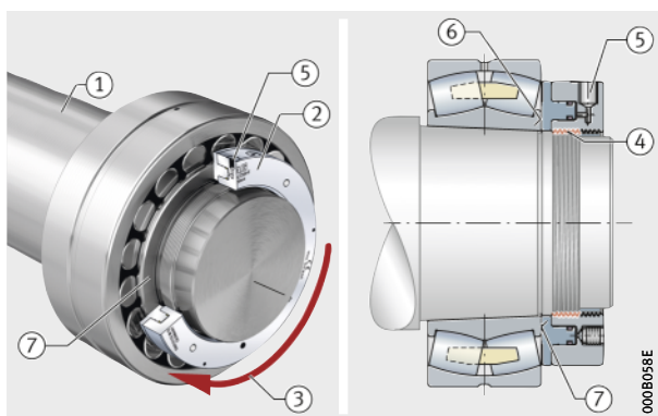
Figura 15 Montaje
