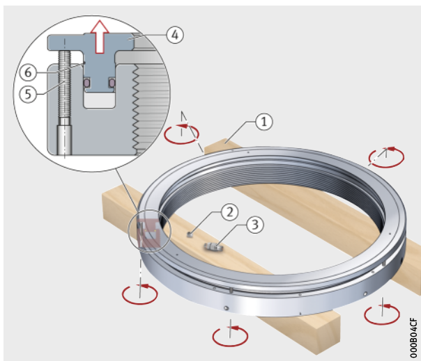
Figura 41 Extracción del cilindro anular
