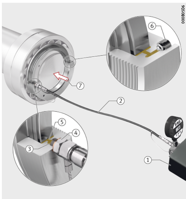
Figura 6 Funcionamiento
